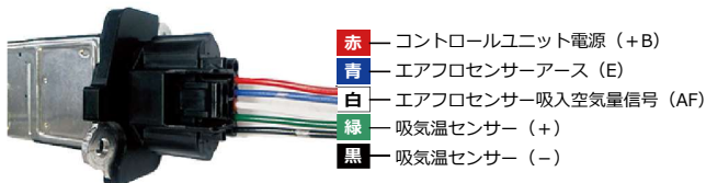
R35 エアフロセンサー (日産純正部品 # 22680-7S00A)
