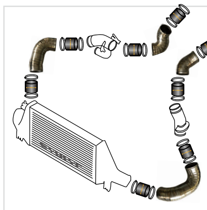
EVOLVE チタンレイアウト (弊社別売インタークーラー取付例)
