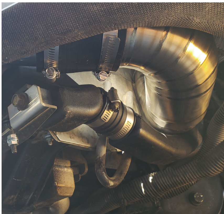
EVOLVE チタンレイアウト (弊社別売インタークーラー取付例)
